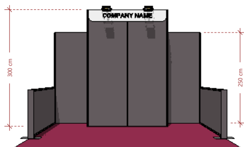
Prospetto un lato aperto | View one open side*
